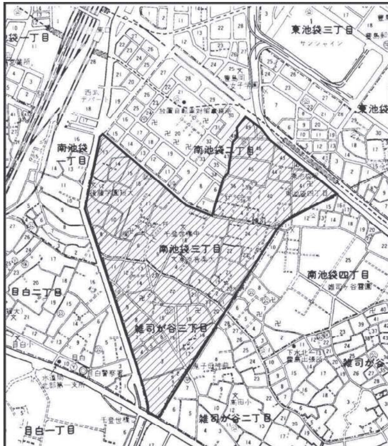
図表 2-3-23 防災生活圈促進事業対象区域図(南池袋地区)
