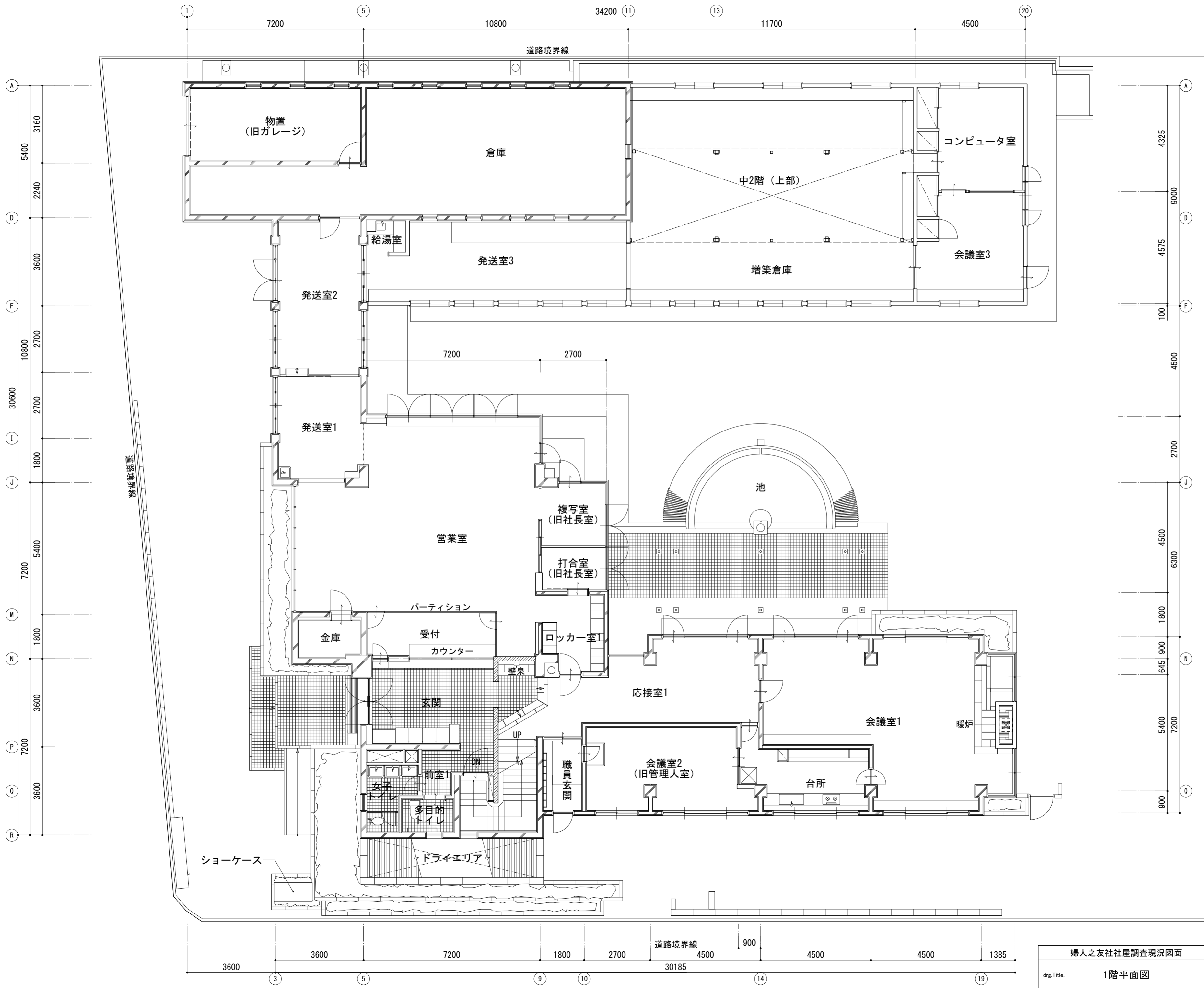
1階平面図
