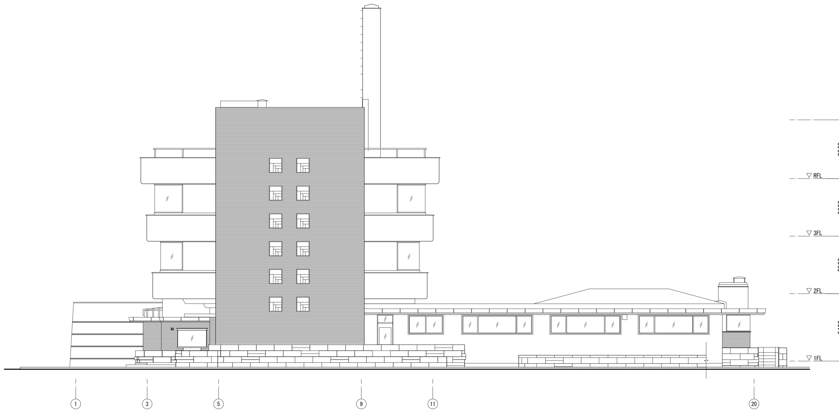
北立面图
