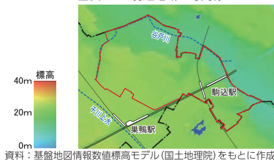
図表5-3 駒込地域の等高線
