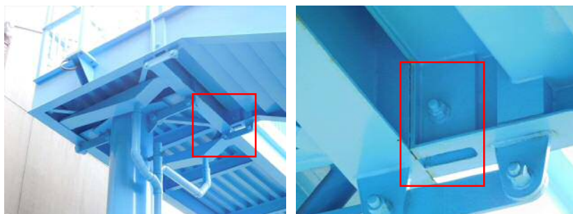
池袋本町四丁目歩道橋 フック部
