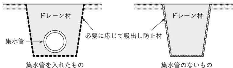
図 3-68 地下排水工の断面
