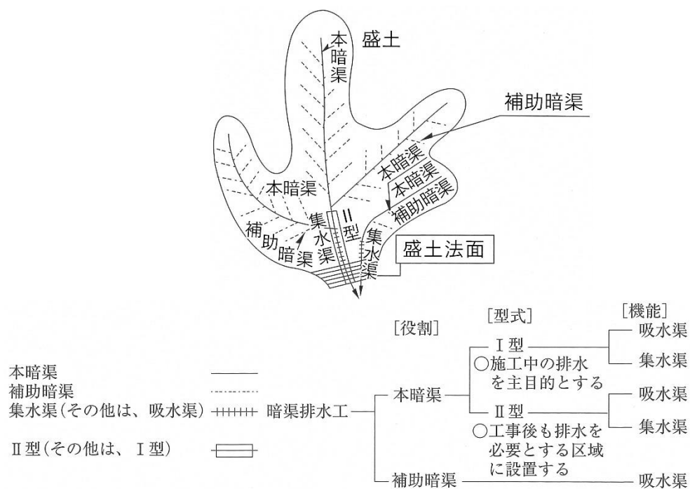
図 3-69 地下水排水工の配置
