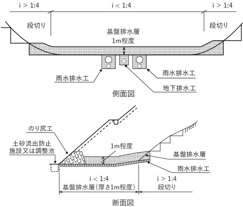
図 3-70 基盤排水層
