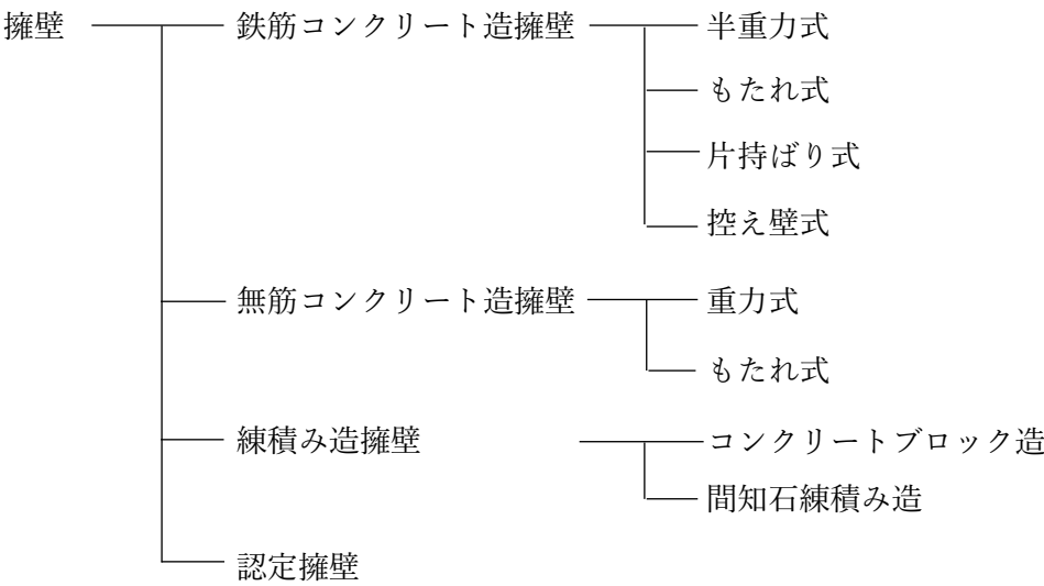
図 3-12 擁壁の種類
