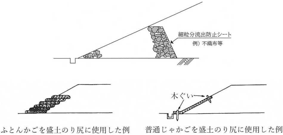
図 3-71 法尻工の例
