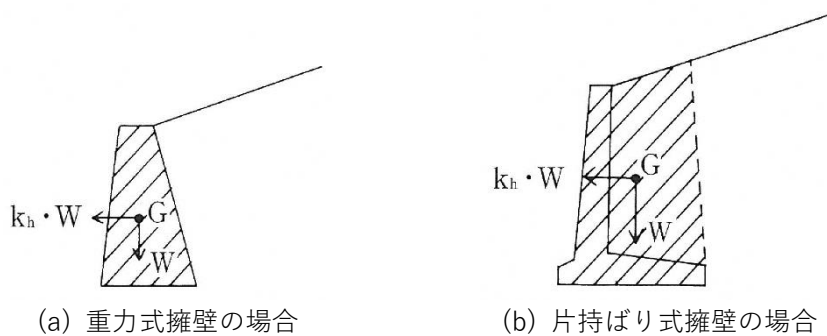
図 3-36 地震時慣性力の考え方
