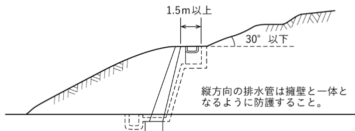
図 3-64 法肩排水工
