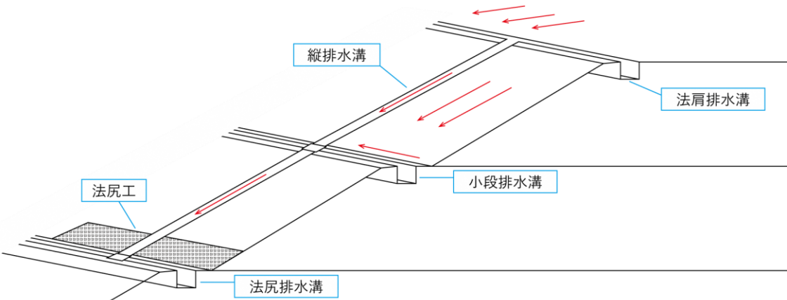
図 3-62 表面排水工の種類
