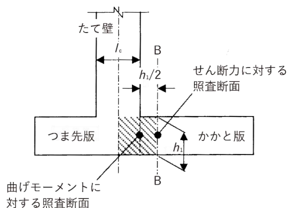
図 3-44 かかと版のせん断力を照査する断面
