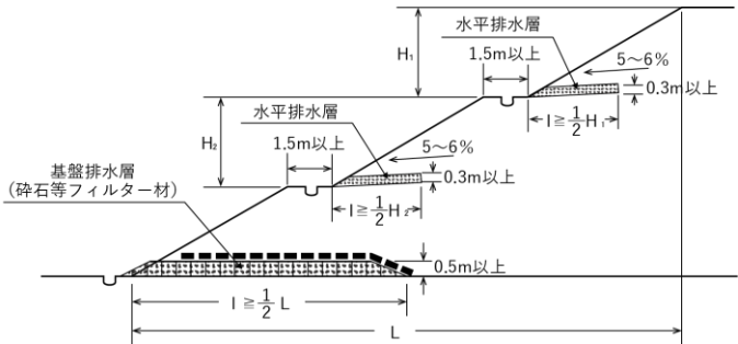
図 3-73 水平排水層
