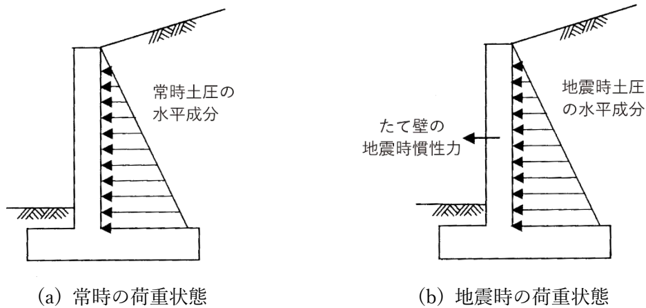
図 3-40 縦壁の断面計算における荷重状態
