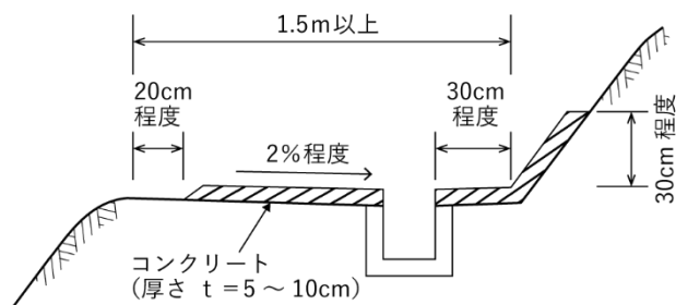
図 3-65 小段排水工
