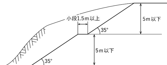
図 3-9 切土法面の形状
