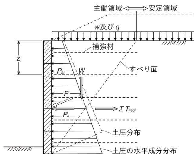
図 3-50 補強土壁自体の安定性の照査に用いる土圧
