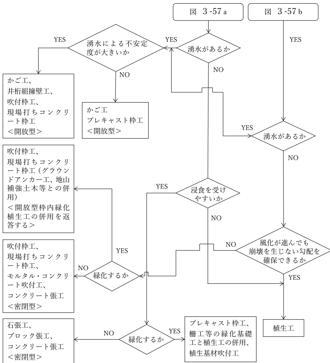
図 3-59 法面保護工の選定フロー③（切土法面の場合）[引用]道路土工 切土・斜面安定工指針（平成21年度版）、一部加工
