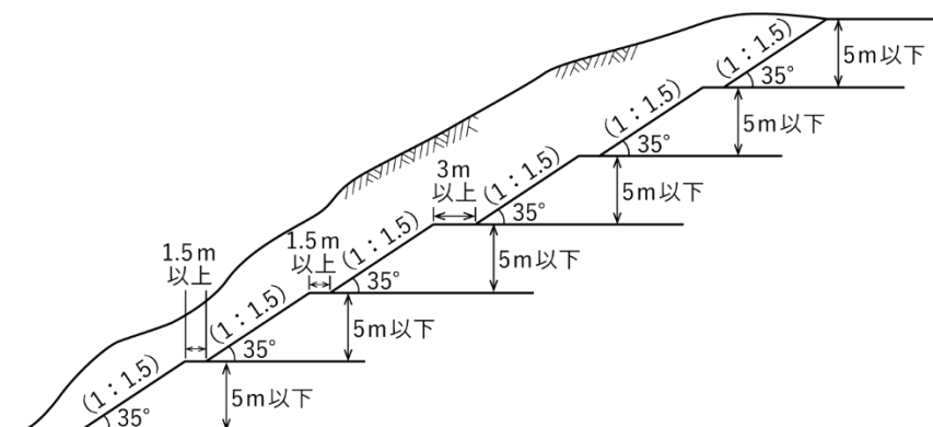
長大法の形状
