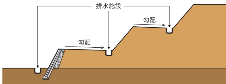
図 3-55 崖面天端の勾配
