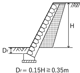
図 3-17 根入れ深さの考え方
