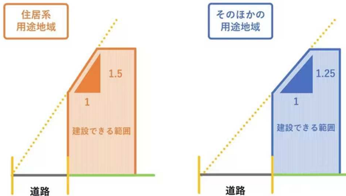
〔図表1〕 道路斜線制限のイメージ
