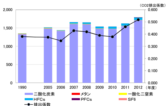
◆温室効果ガス排出量の推移
