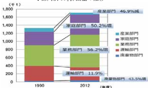
◆部門別CO 2 排出量の推移
